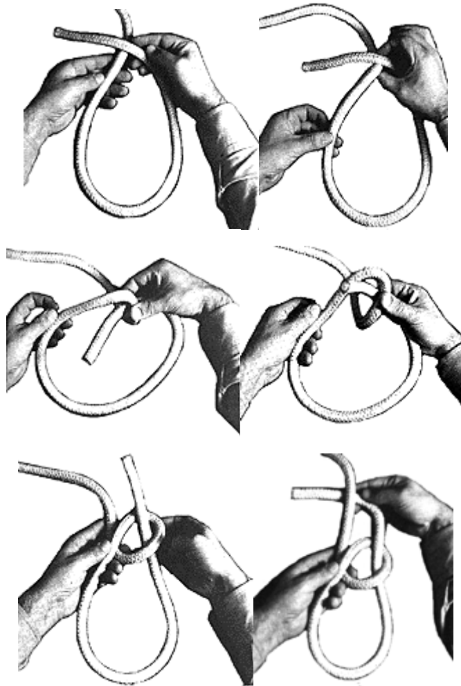
Esecuzione della gassa d'amante (Metodo delle due dita)
