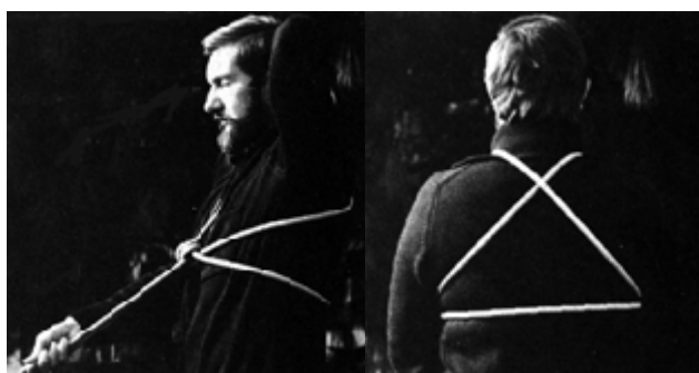
Cintura di sicurezza a esecuzione ultimata
